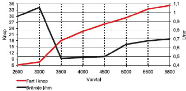
FART OCH BRÄNSLEFÖRBRUKNING (2 pers) HR 480 SC, SUZUKI DF70A
