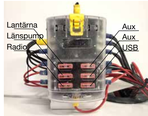
Säkringsbox, som är placerad under instrumentpanelen på båda modellerna.
