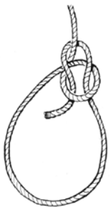
Pålstek.
